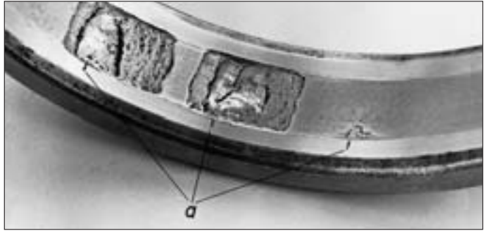
110: Vorzeitige Ermüdung bei einem Zylinderrollenlager-Außenring als Folge von Schürfmacken, die bei „a“ noch zu erkennen sind
