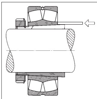
90: Ausbau eines kleinen Pendelrollenlagers mit Spannhülse. Mit Hilfe eines Metalldorns treibt man den Innenring von der Hülse.
