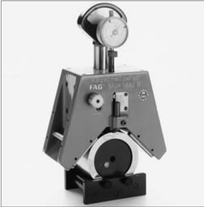
12: Das Kegelmessgerät FAG MGK 132 eignet sich für Kegellängen ab 80 mm und Kegeldurchmesser von 90 bis 820 mm.
