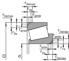
Kegelrollenlager
