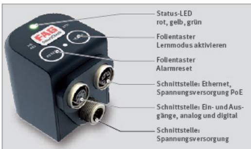
Bedienelemente und Schnittstellen des FAG SmartCheck
